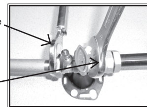
Raccordement sortie rob type E et E1
