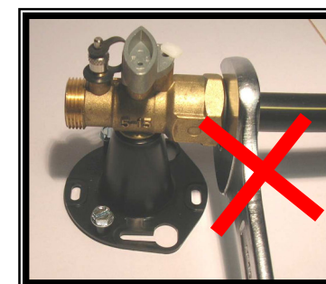
Raccordement sortie rob type E et E1
