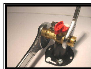
Raccordement sortie rob type E et E1
